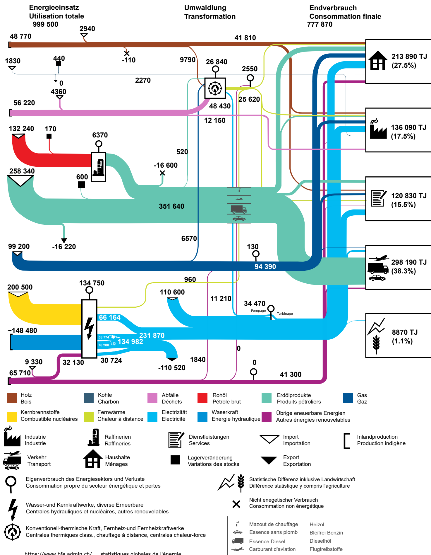
Fig. 5 Detailliertes Energieflussdiagramm des Schweiz 2025 (in TJ) Flux énergétique détaillé de la Suisse en 2025 (en TJ)
